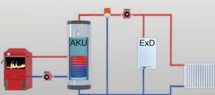
Schéma zapojení 3
