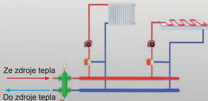
Schéma zapojení 4
