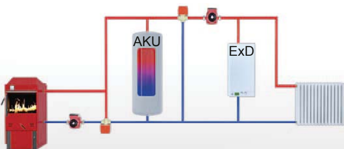
Schéma zapojení 1
