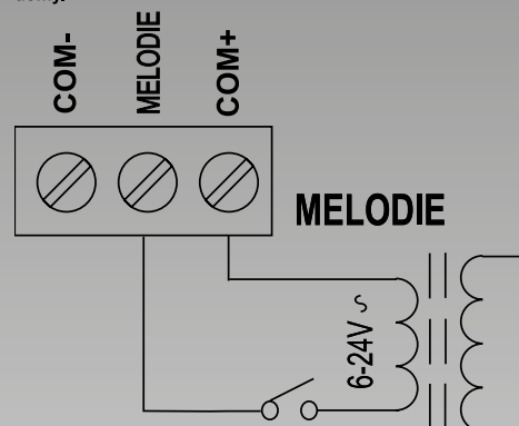
Schéma č.2 - Zapojení pro ovládání střídavým napětím 6-24V~, např. pro panelové domy.
