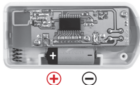
Obr.6 Polarita batérie
